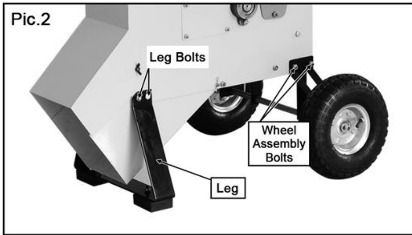
Pic.2 Fixation de la jambe
